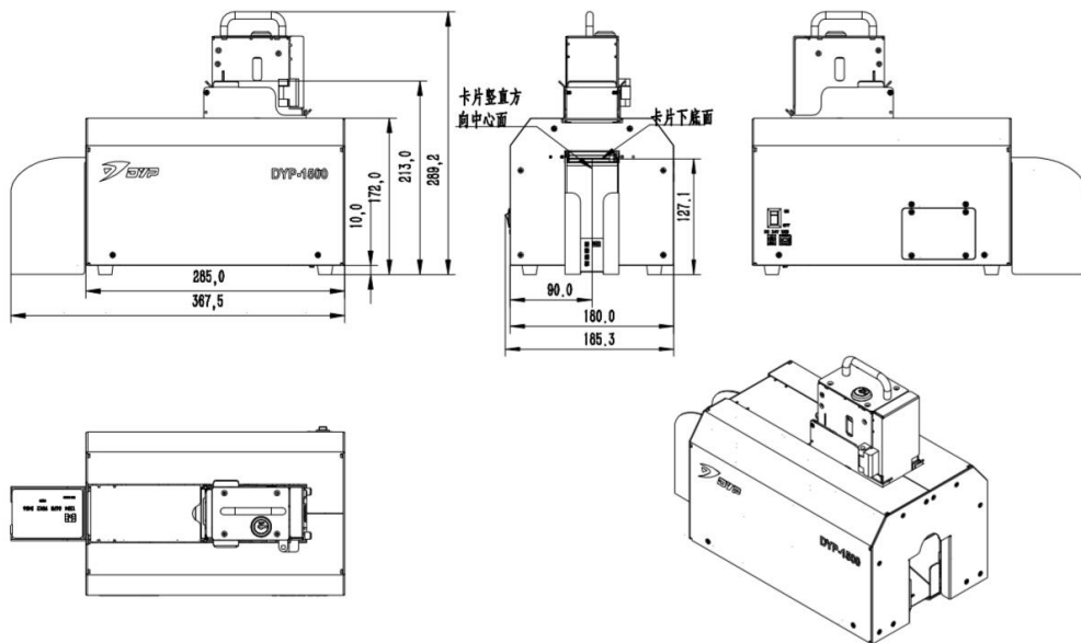
DYP-1500尺寸图
